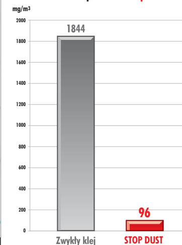
Poziom koncentracji pyłu w zwykłym kleju oraz w kleju CM17 StopDust
